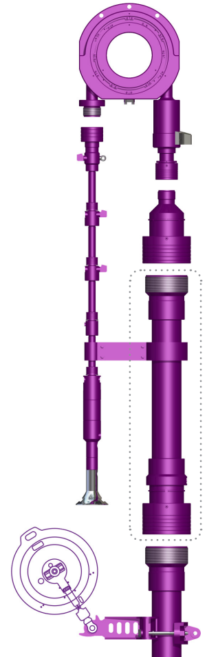
Wireline PCE Stack
